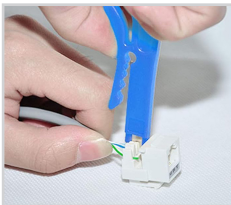
(Punch Down Action)
